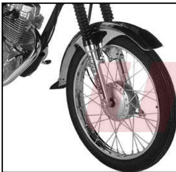
Rueda delantera con freno de tambor a expansión interna
